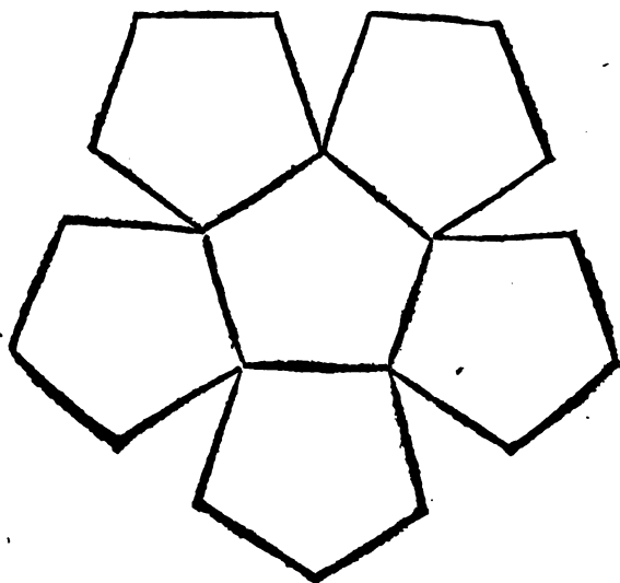
Duodecedron.
