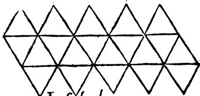
Icosa hedron.
