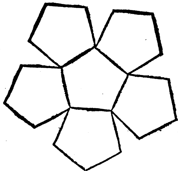
Duodecedron.
