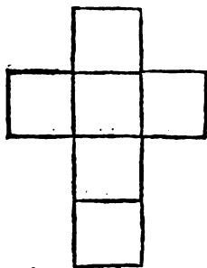
Hexacedron.
