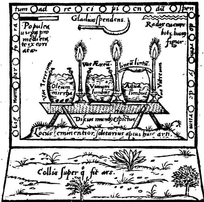
Planum Terra.
