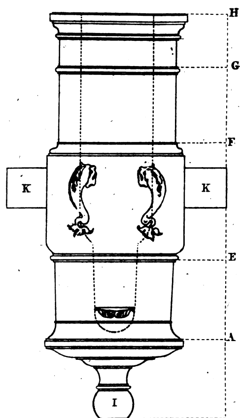
HOWITZ Fig. 11.
