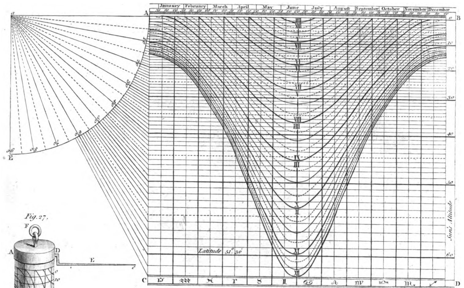
Portable D I A L.
