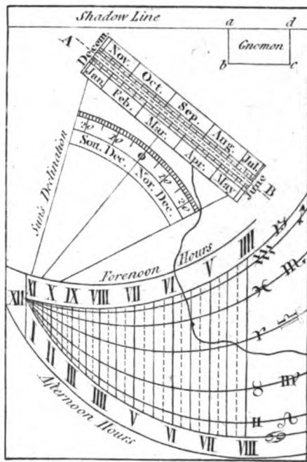
Portable D I A L.
