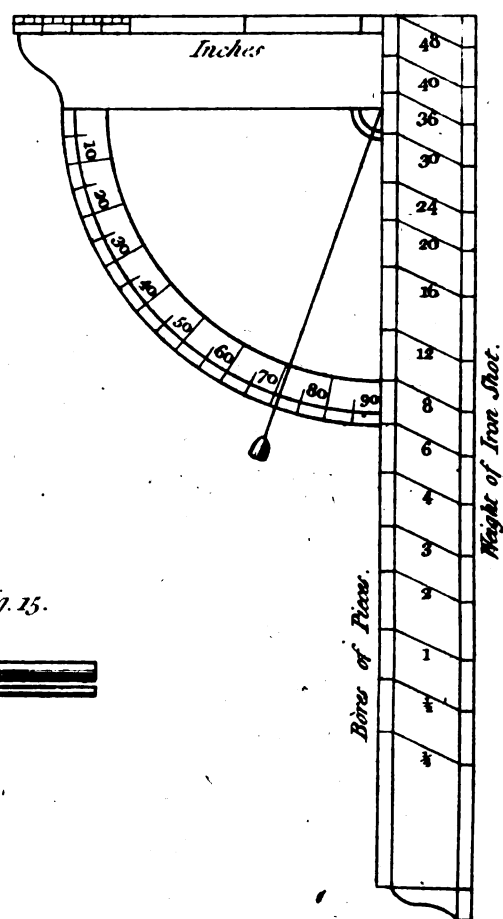
QUADRANT Fig. 14
