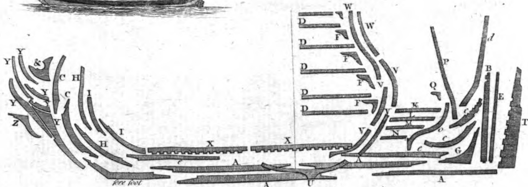
Elevation Fig. 6.
