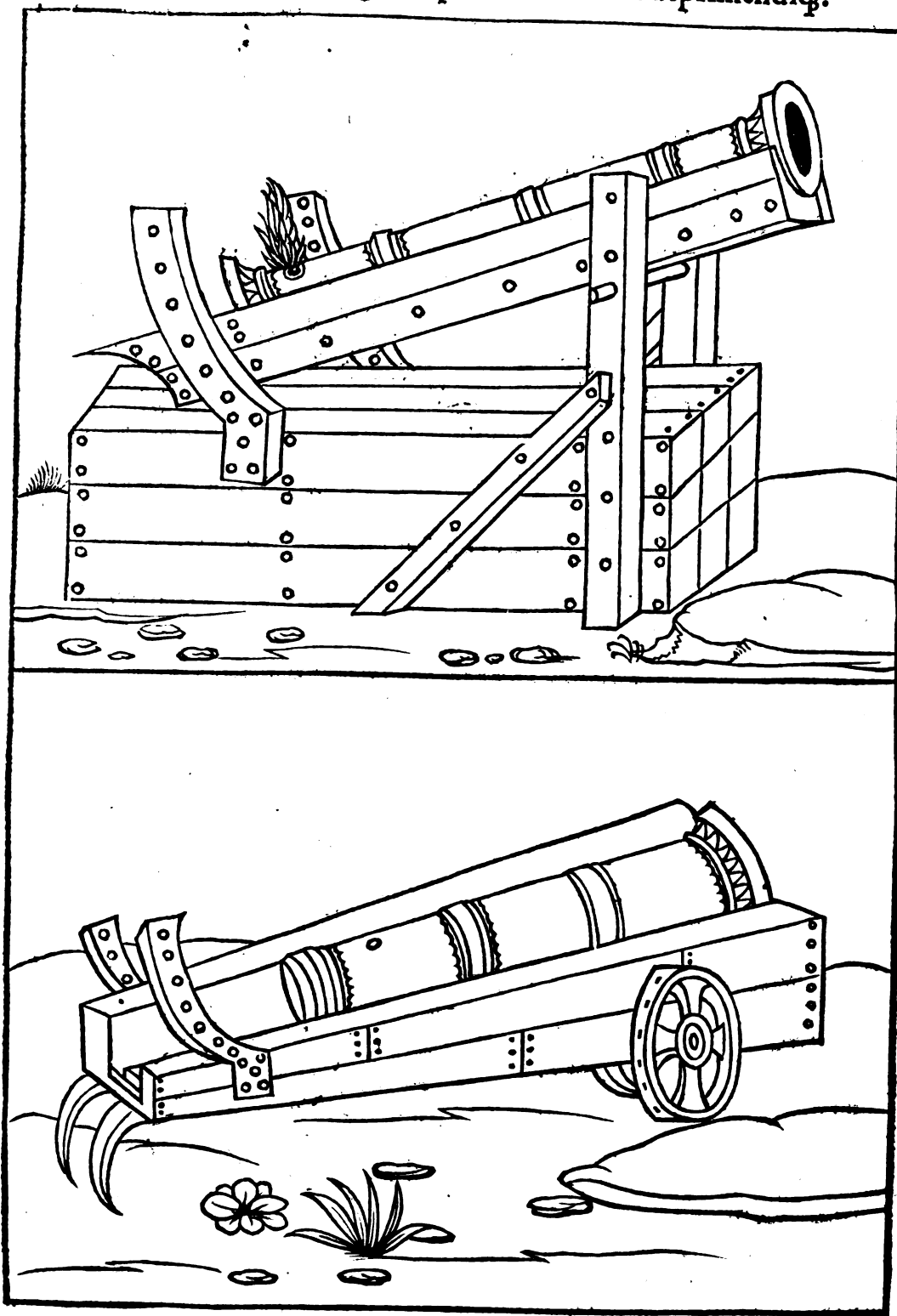
Instrumentum ad tormenta deprimenda extollendâque.
