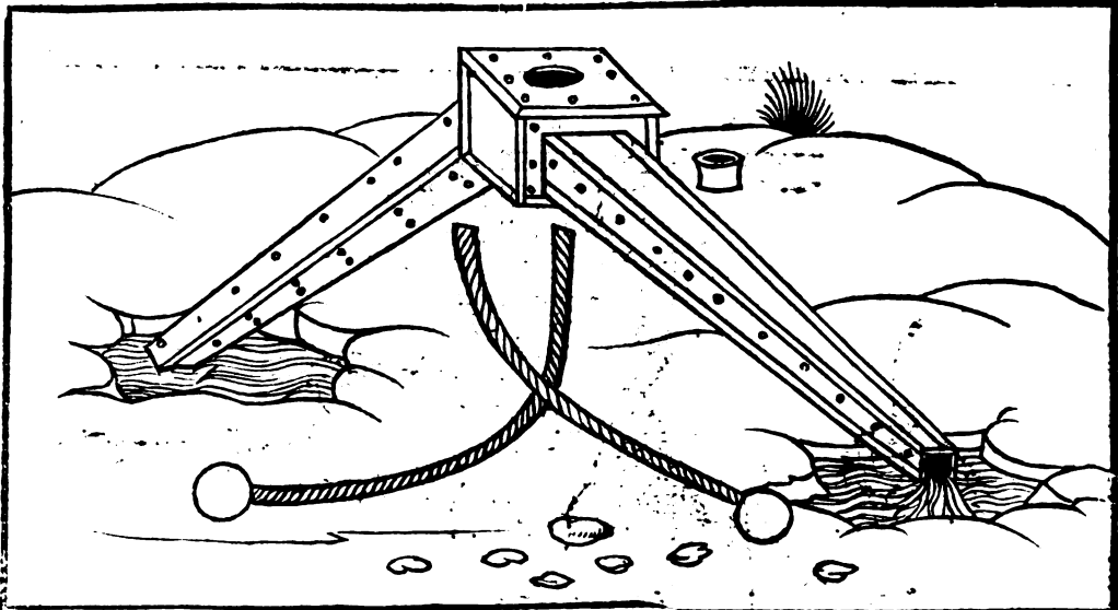
Aliud educendi aquam instrumentum.
