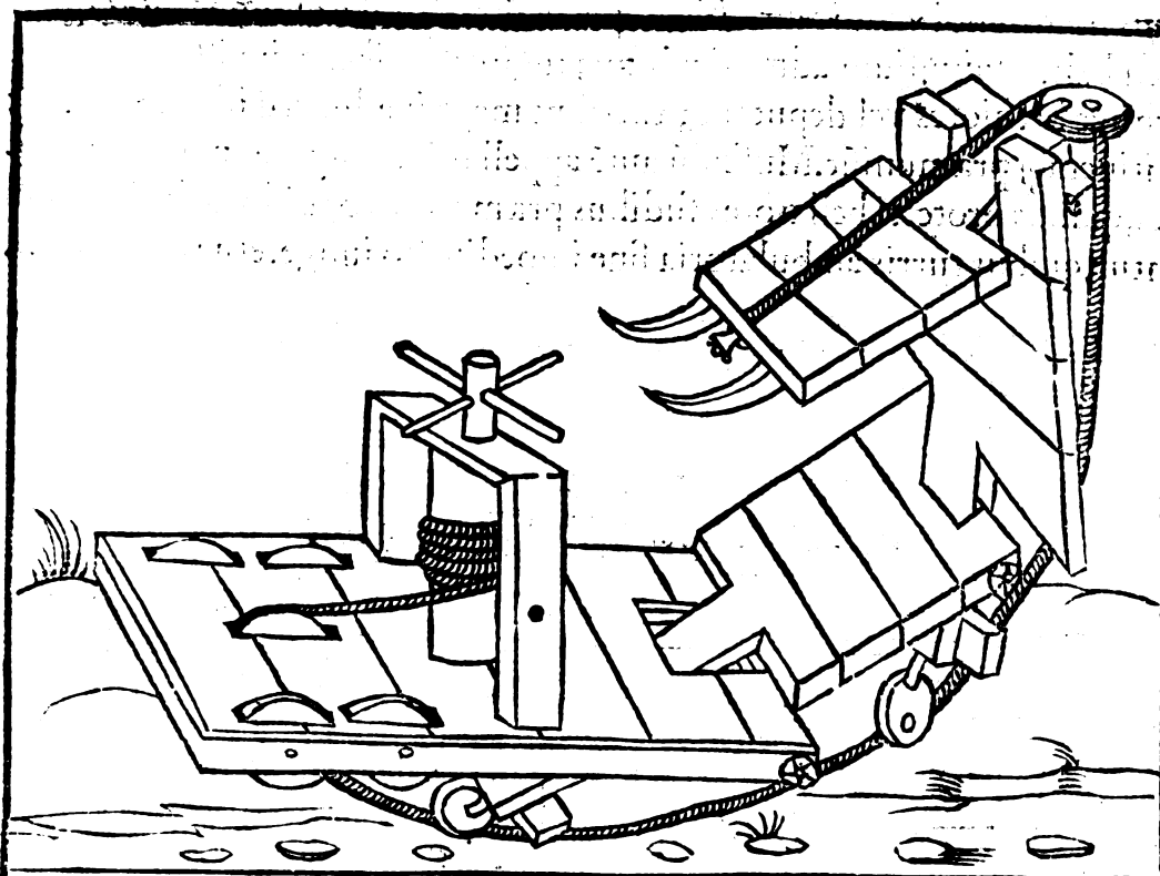
Producendi pontis instrumentum.
