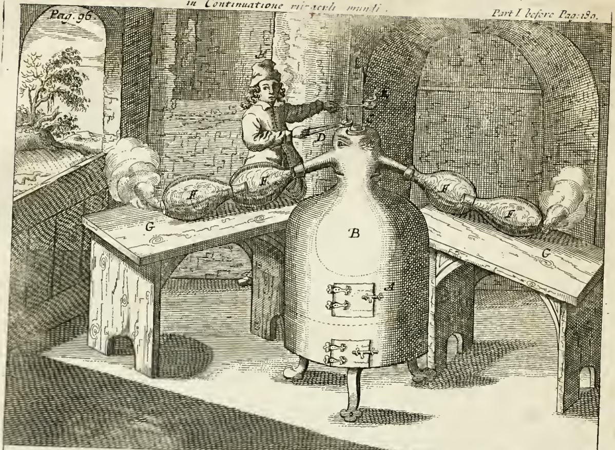
A. Ist der Ofen. B. Das distillier gefäs in dem Ofen. C. Das loch mit einem fultz dar durch das swänge eingetrag wird. D. Die Zänge mit deckel dar mit das F. Die recipienten. E. Ein Eysen löffel dar mit der schwin eingetrag wird. F. Die bank darauf die recipienten liegen. G. der Laborant.
