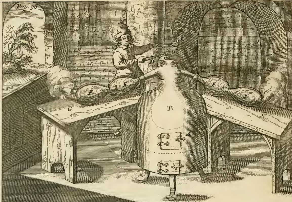
A. Ist der Ofen. Das swärze eingetragen wird. B. Ein Eysen löffel dar mit der schwan eingetragen wird. B. Das distillier gefäs in dem Ofen. D. Die Zange mit lockel dar mit das F. Die reapiemen. G. Die bank dar auf die reapiemen. C. Das löch mit einem falz dar durch gefäs nach dem ein tragen geschloffe wird: unten hyn. H. der Laborant.
