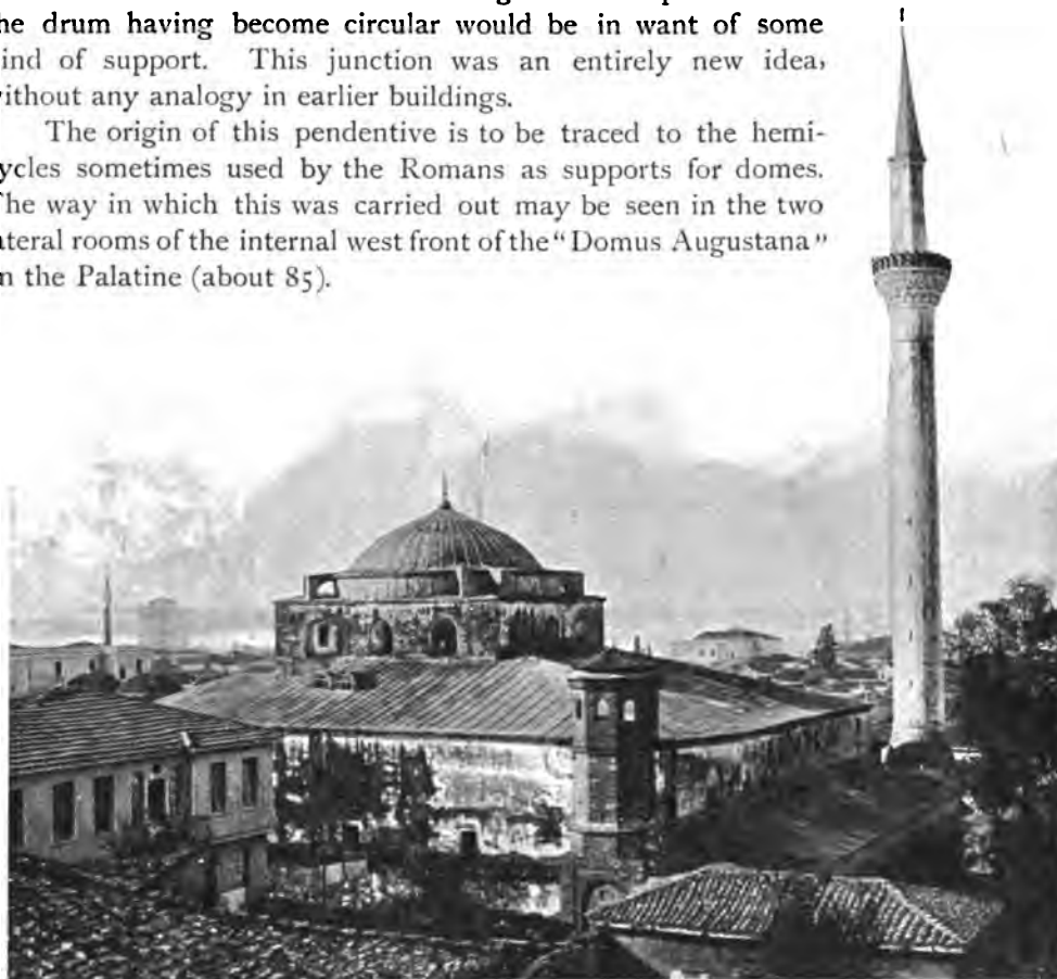
Fig. 110.—Salonica. St. Sophia (about 425).
