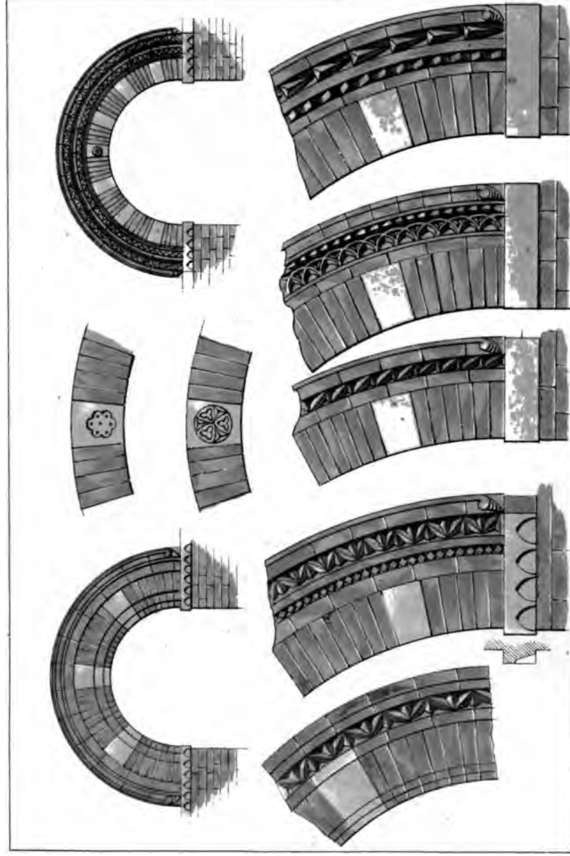
BROLETTO - BRESCIA. Details of Archivolts.
