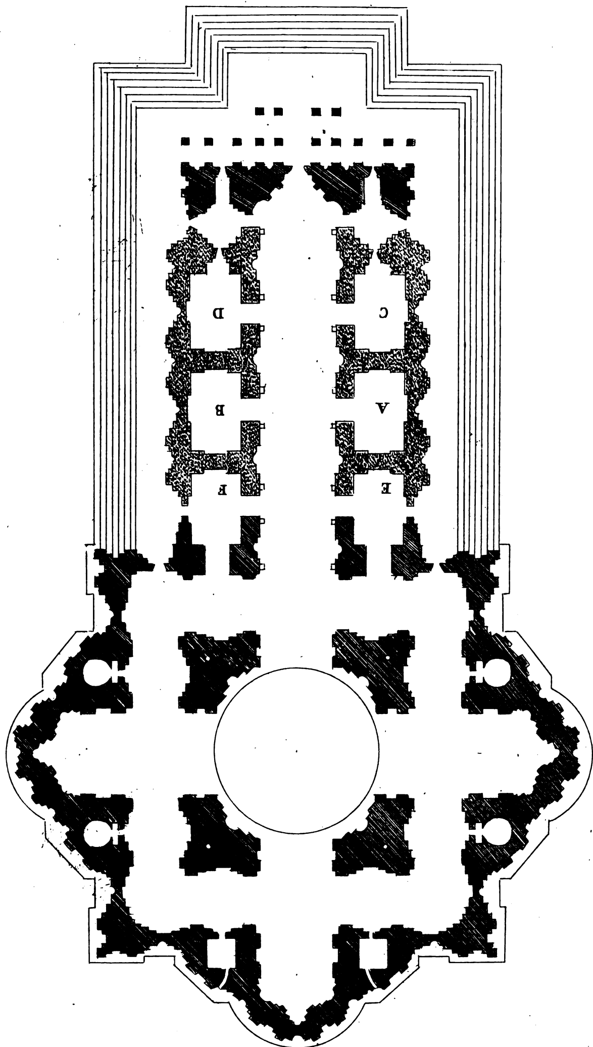
ICHOGRAPHIA TEMPLI A BONAROTA DELINEATI CVM ADDITAMENTO INCEPTO SVB PAVLO V.
