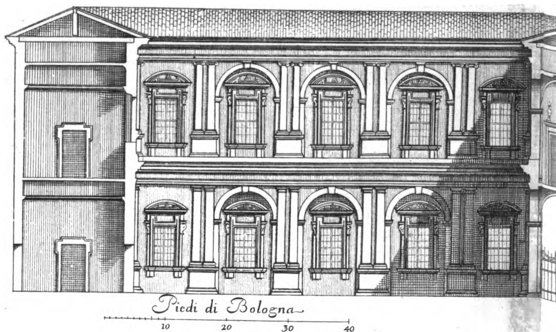
Spaccato del Palazzo dell'Istituto delle Scienze
