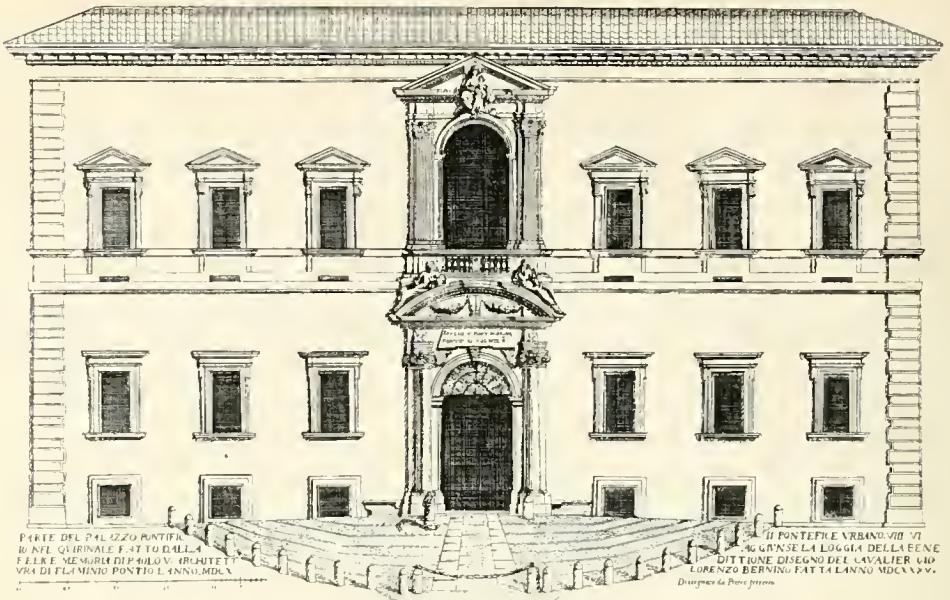
Abb. 13. Fassade des Palazzo del Quirinale mit der Loggia Berninis. Nach Ferrerio, Palazzi di Roma.
