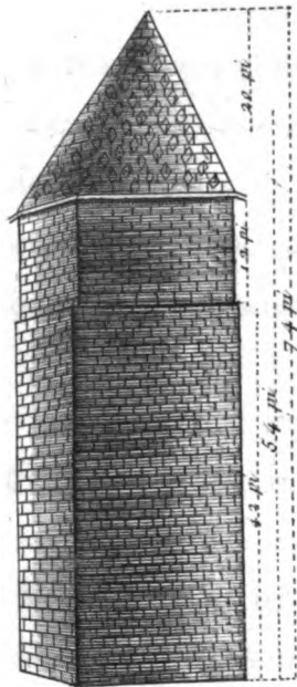
Plan de la Pile de Pirrelonge.
