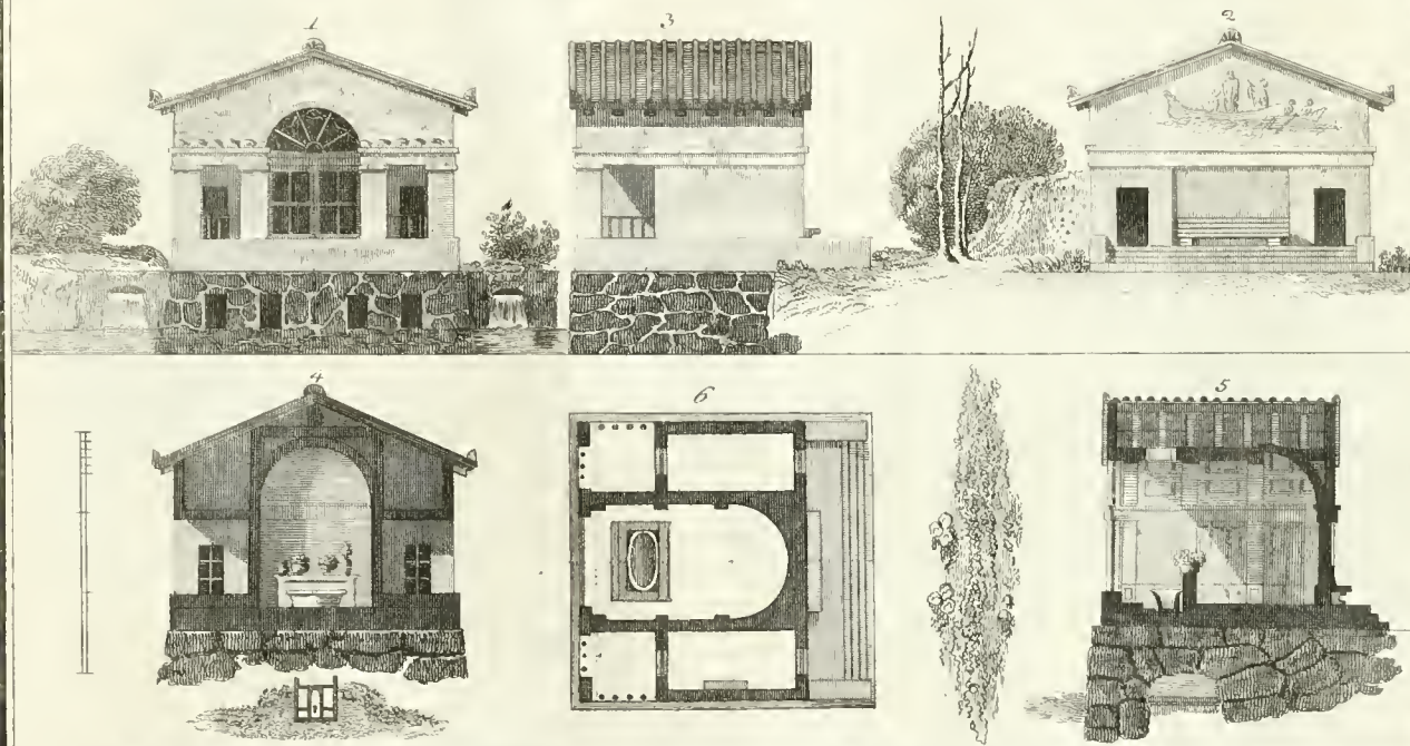
Antica fabbrica per uso de' bagni 1 Prospetto principale 2 Prospetto opposto 3 Parte laterale 4 Spaccato 5 Altro spaccato per traverso 6 Pianta generale
