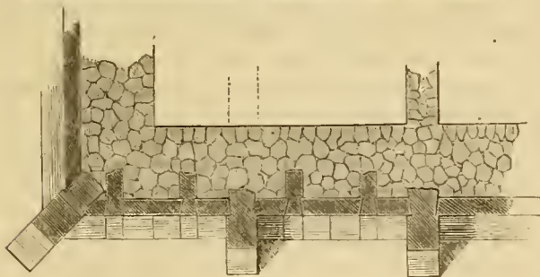
Unterbau des Olympiums zu Athen. (Eigene Aufnahme.)
