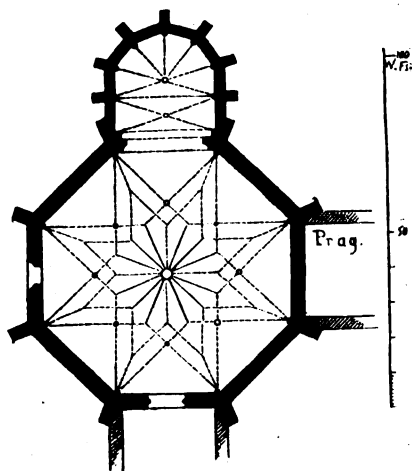
Grundriss der Karlsrufer Kirche zu Prag. (Nach Grueber.)
