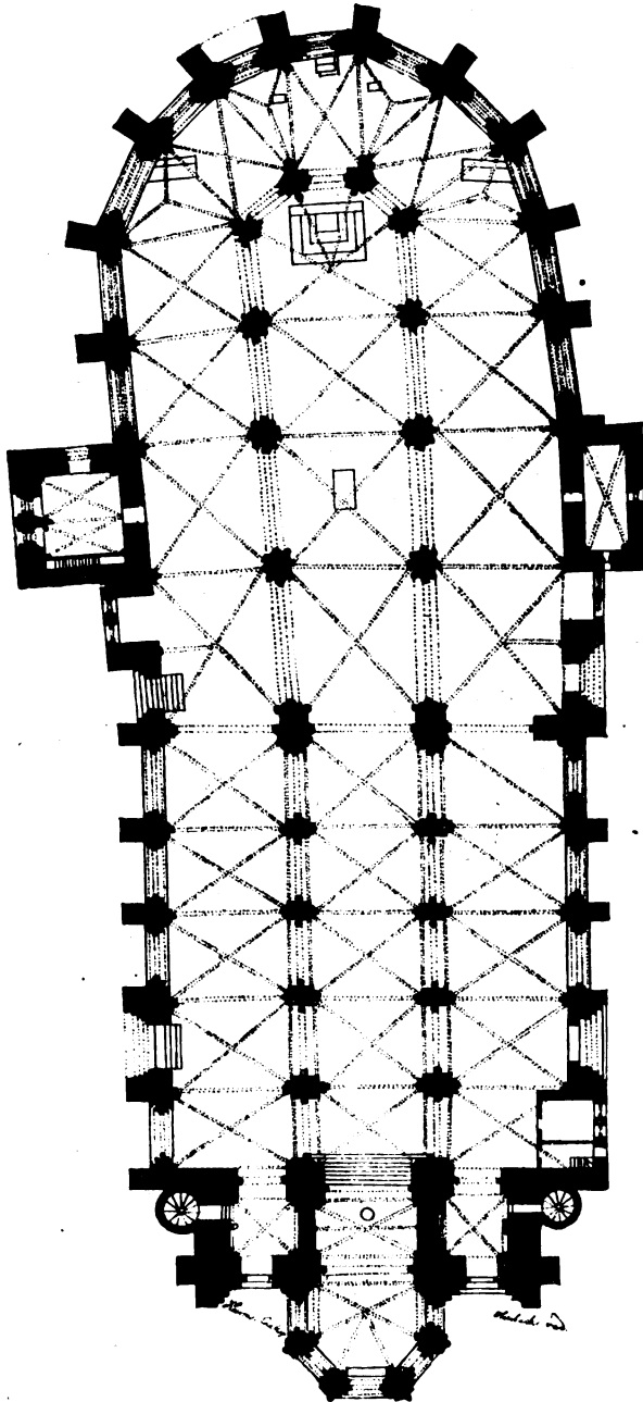
Grundriss der Sebalduskirche zu Nürnberg. (Aus Rettberg, Nürnbergs Kunstleben.)
