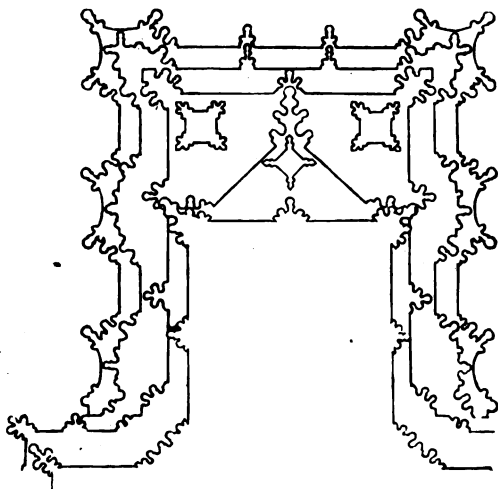
Dom von Köln. Profil des Gliederwechsels an den Hauptstrebenpfeilern des Thurmbaues im zweiten und dritten Geschoss. (Nach Boissérée.)
