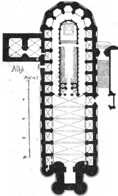
Grundriss der Kathedrale von Alby. (Nach Chapuy.)
