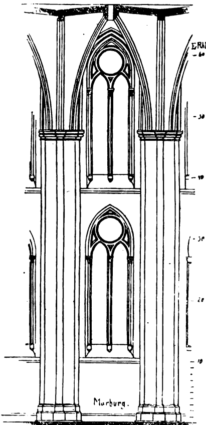
Elisabethkirche zu Marburg. Inneres System. (Nach Moller.)
