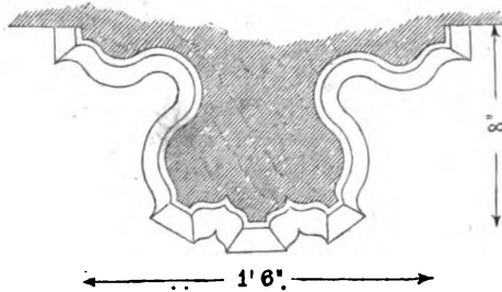
Wänddienst im Chor der St. Veitskirche von Mühlhausen. (Aus der Kunst des Mittelalters in Schwaben.)
