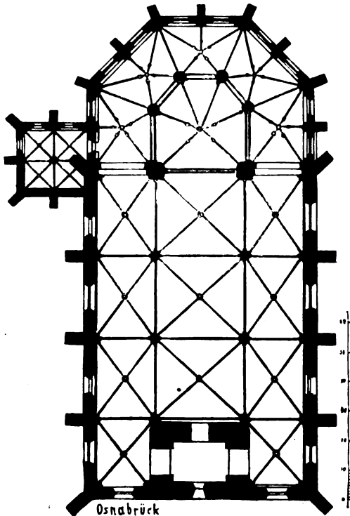
Grundriss der Marienkirche zu Osnabrück. (Nach Lübke.)
