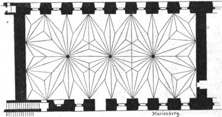
Grundriss des Conventremters auf Schloss Marienburg. (Nach Rabe.)
