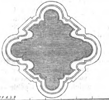
Profil der Hauptpfeiler im Schiff der Marienkirche zu Mühlhausen. (Nach Puttrich.)
