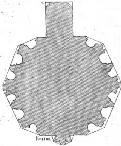
Dom zu Krakau. (Profil der Schifffpfeiler. (Nach Essenwein.)
