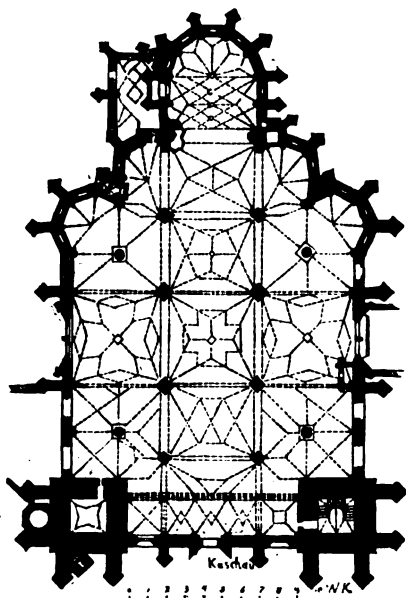
Grundriss des Domes zu Kaschau. (Nach Henszlmann.)
