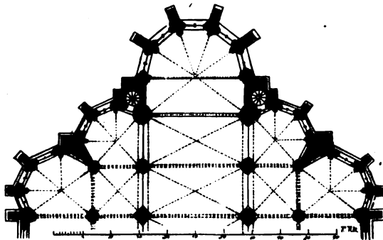
Chorhaupt des Domes von Xanten. (Nach Schimmel.)
