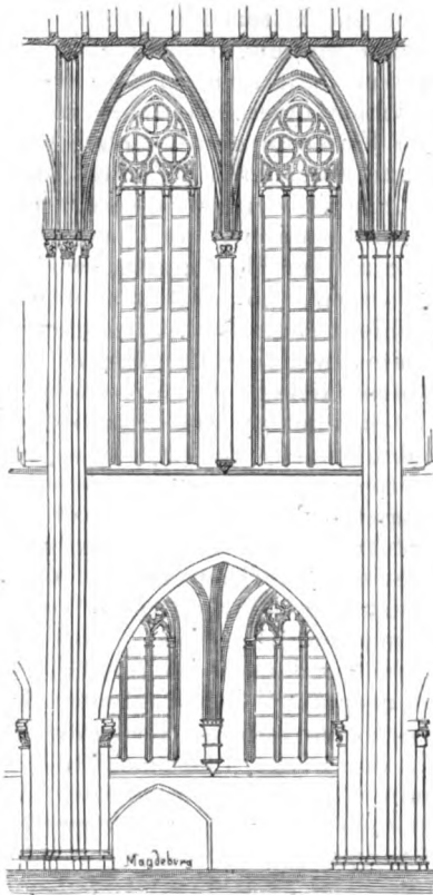
System im Schiffbau des Doms von Magdeburg. (Nach Clemens Mellin und Rosenthal.)
