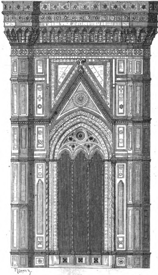
Obergeschoss des Domthurmes von Florenz. (Nach Runge.)
