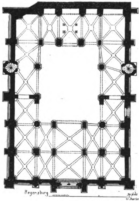
Grundriss der alten Pfarr in Regensburg. (Nach Popp und Balau.)
