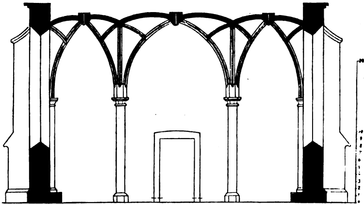
Querschnitt der Schwanenkirche bei Forst. (Nach Reichenesperger.)
