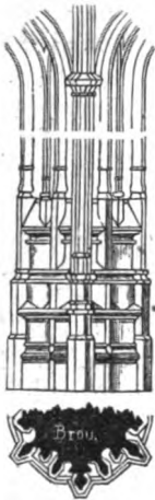
Kirche zu Brou. System der Pfeilergliederung. (Nach Peyré.)
