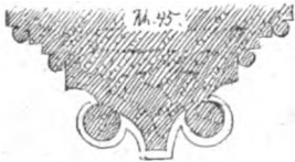
Quergurtprofil im Schiffgewölbe von St. Maria auf dem Kapitol zu Köln. (F. K.).
