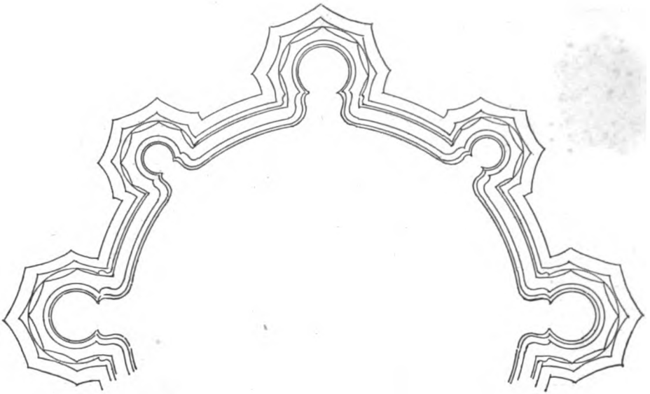
Stiftskirche zu Wetzelar. Grundriss des nördlichen Kreuzpfellers. (F. K.)
