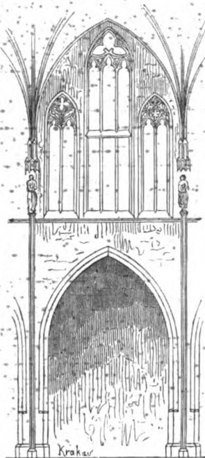
Dom zu Krakau. — inneres System des Schiffes. (Nach Essenwein.)
