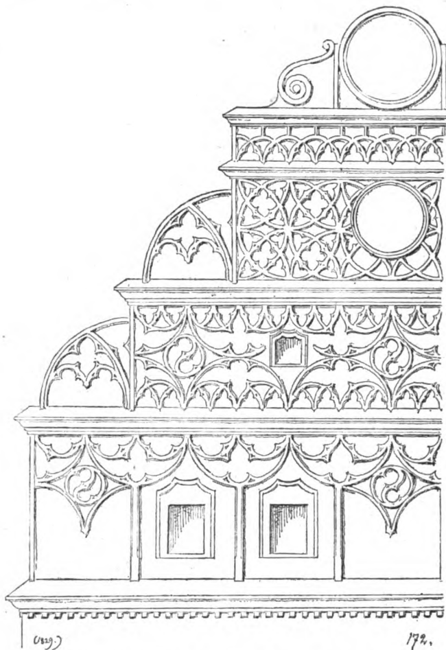
Giebeldekoration des Rathhauses zu Stargard. (F. K.)
