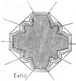
Profil der Schiffpfeiler in der Petrikerche zu Görlitz. (Nach Puttrich.)
