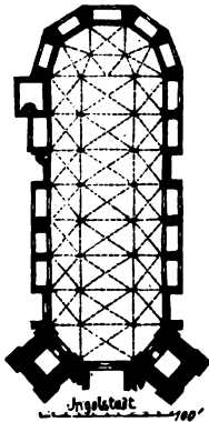
Grundriss der Frauenkirche zu Ingolstadt. (Nach Wiebeking.)
