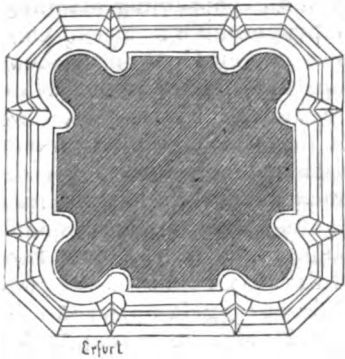
Profil der Mittelschiffpfeiler in der Severikirche zu Erfurt. (Nach Kallenbach.)
