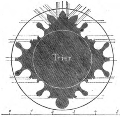
Dienst- Bogen- und Rippenprofile über den Säulen der Liebfrauenkirche zu Trier. (Nach Ch. W. Schmidt.)
