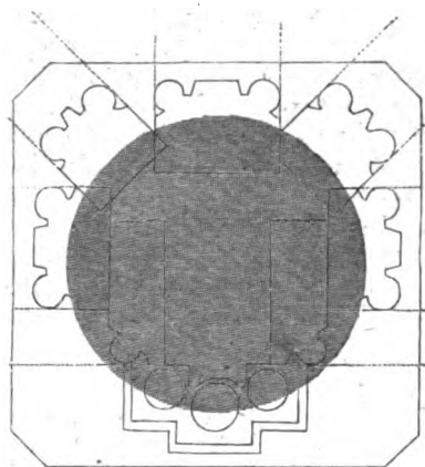
Kathedrale von Paris. Profil der Schiffsäule und der darüber aufsetzenden Bögen, Gurte, Rippen und Dienste. (Nach Viollet-le-Duc.)
