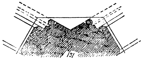
Gertrudskirche bei Rügenwalde. Profil der Bogengliederungen im Mittelraum. (F. K.)
