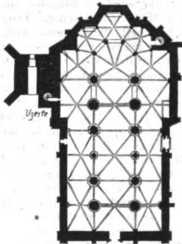
Grundriss der Kirche von Uzeste. (Nach Parker.)
