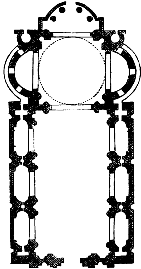
Fig. 90. Grundriss der Kirche Il Redemptore zu Venedig.
