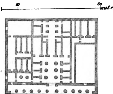
Fig. 27. Tempel von Qurna.
