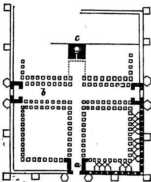
Fig. 52. Grundriss des Palastes zu Salona.
