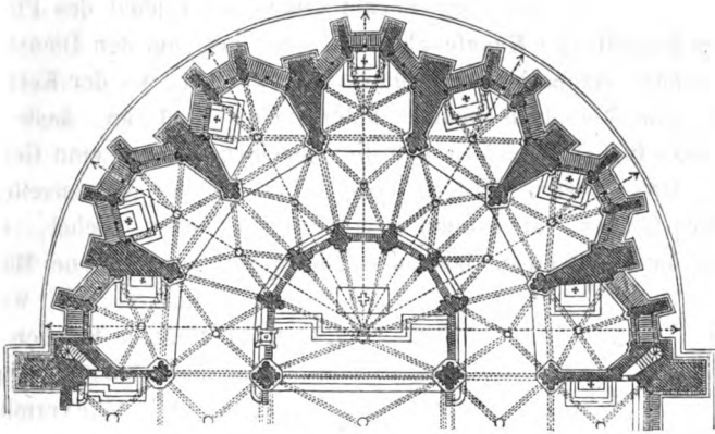
Fig. 78. Chorbaupt vom Kölner Dome.
